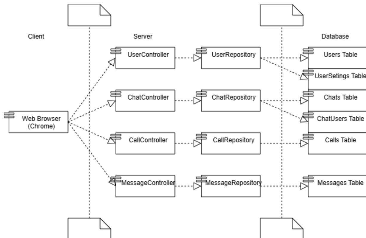
Рис. 2 Концептуальна діаграма компонентів
