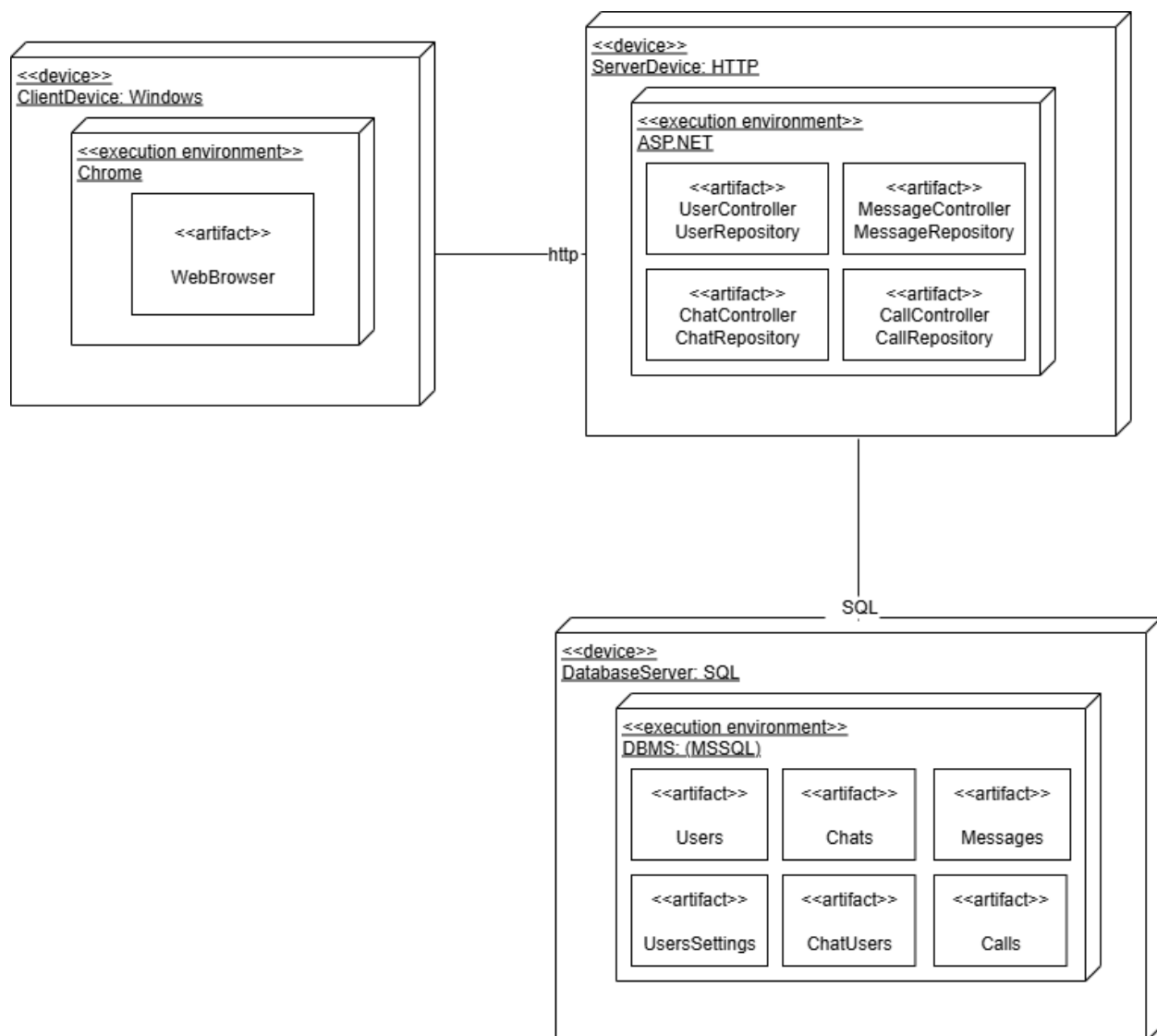
Рис. 3 Діаграма розгортання системи
