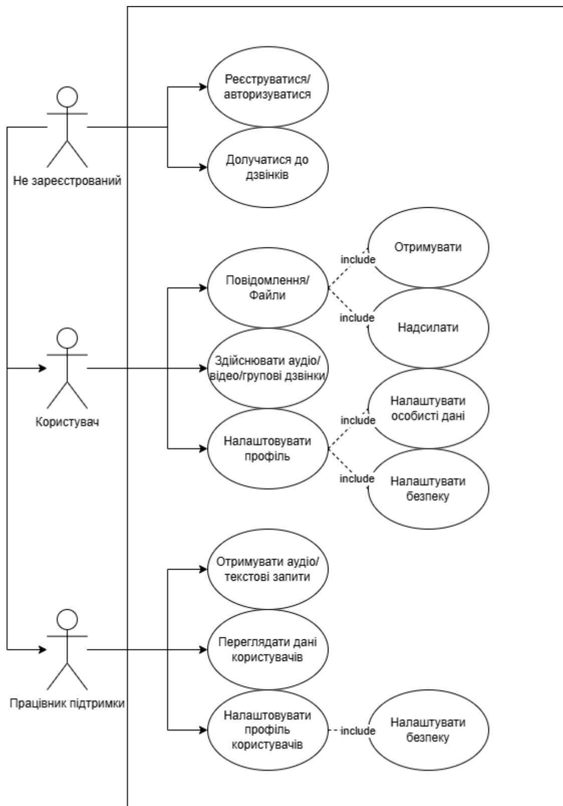
Рис. 1 Діаграма варіантів
